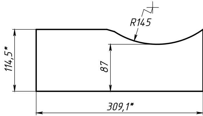
Поз.2 (Угольник)
